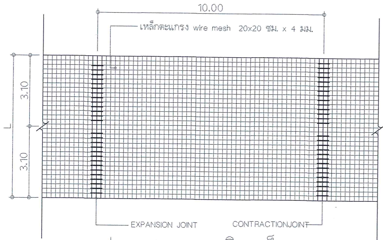
แปลนแสดงการเสริมเหล็กถนน คสล.
