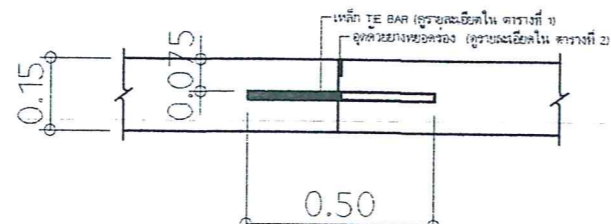
LONGITUDINAL JOINT
