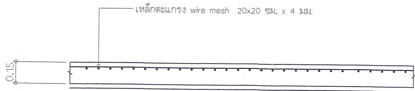
รูปตัดตามยาวเหล็กเสริมคอนกรีต
