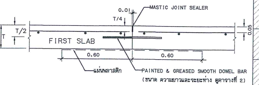
LONGITUDINAL JOINT
